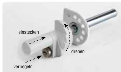
Funktionsweise der Bandsicherung BS1-Z.
