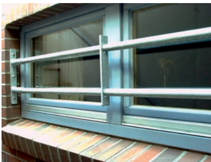
Abb.: Rollstabsicherung Typ RSM-2-200 (Doppelstab Achsmaß 200mm) mit Mittelstrebe RS-M
